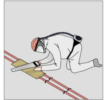
Enrobage des gaines et arasement de l'excédent
