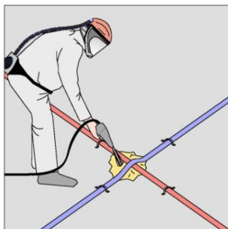
Projection sur les croisements de gaines
