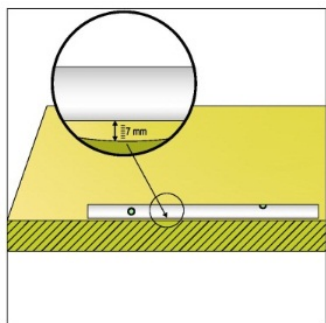
Tolérance de 7 mm sous la règle de 2 m
